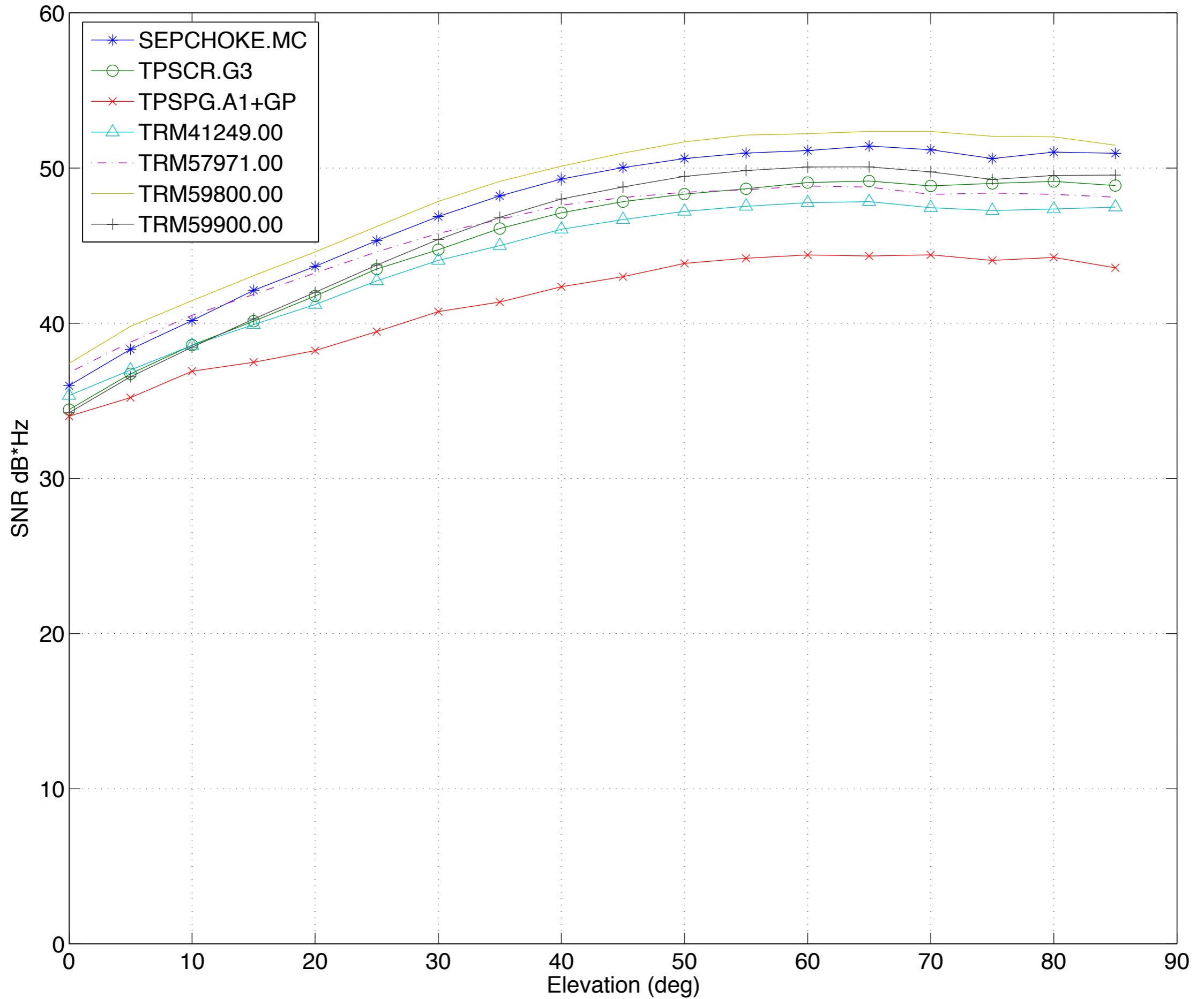
GLONASS L1 SNR
